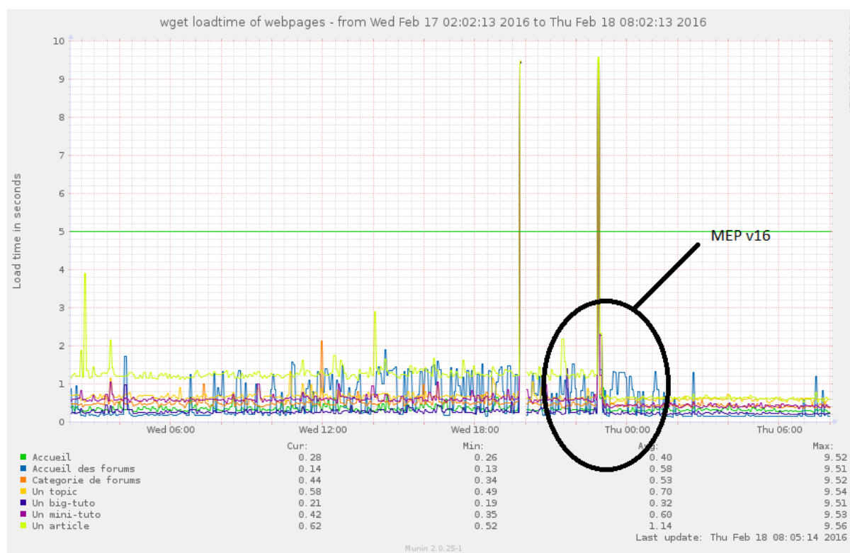
Figure 3.1 – Amélioration significative des performances sur la v16
